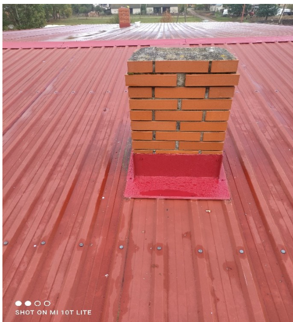
Rysunek 168 naprawa obróbek dekarских dachu remizo-świetlicy
